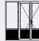
Porte-fenêtre à la française 3 vantaux dont 1 fixe
